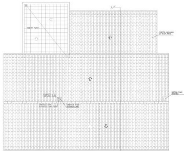
PLANTA COBERTA
