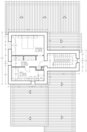
PLANTA PISO SUP. CONSTRUIDA VIVIENDA (POR VOLUMEN) 53,66 M 2 SUP. CONSTRUIDA VIVIENDA (POR ANEXO/ANEXOS) 24,00 M 2
