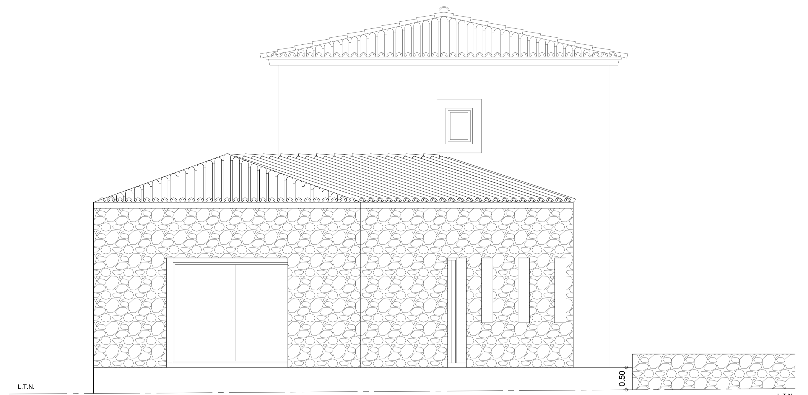
FACHADA LATERAL IZQUIERDA
