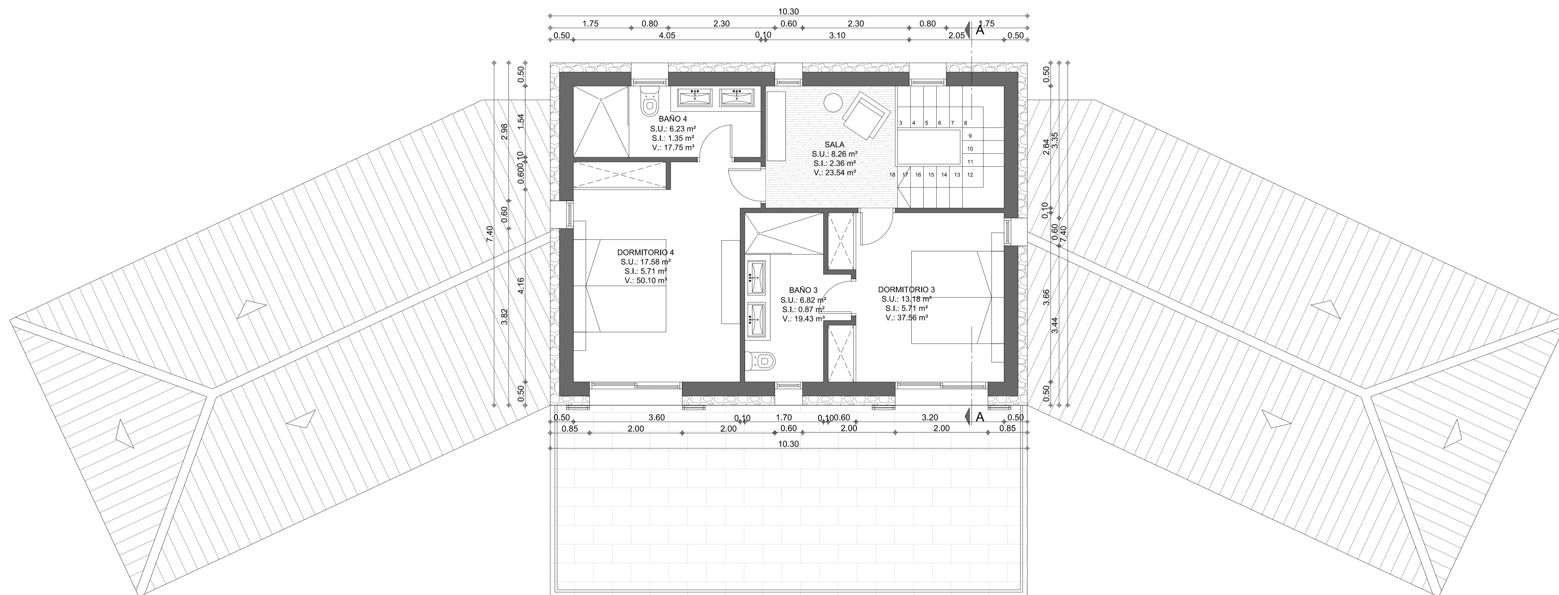
PLANTA PISO
