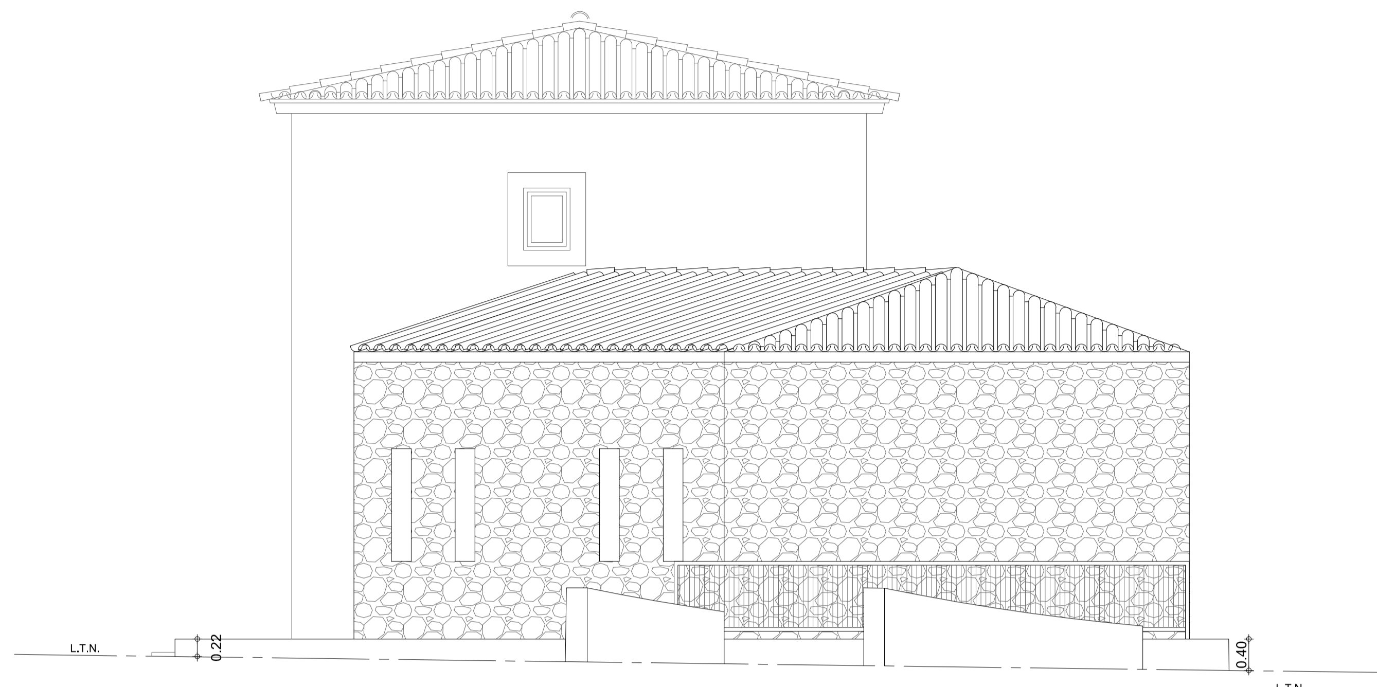
FACHADA LATERAL DERECHA
