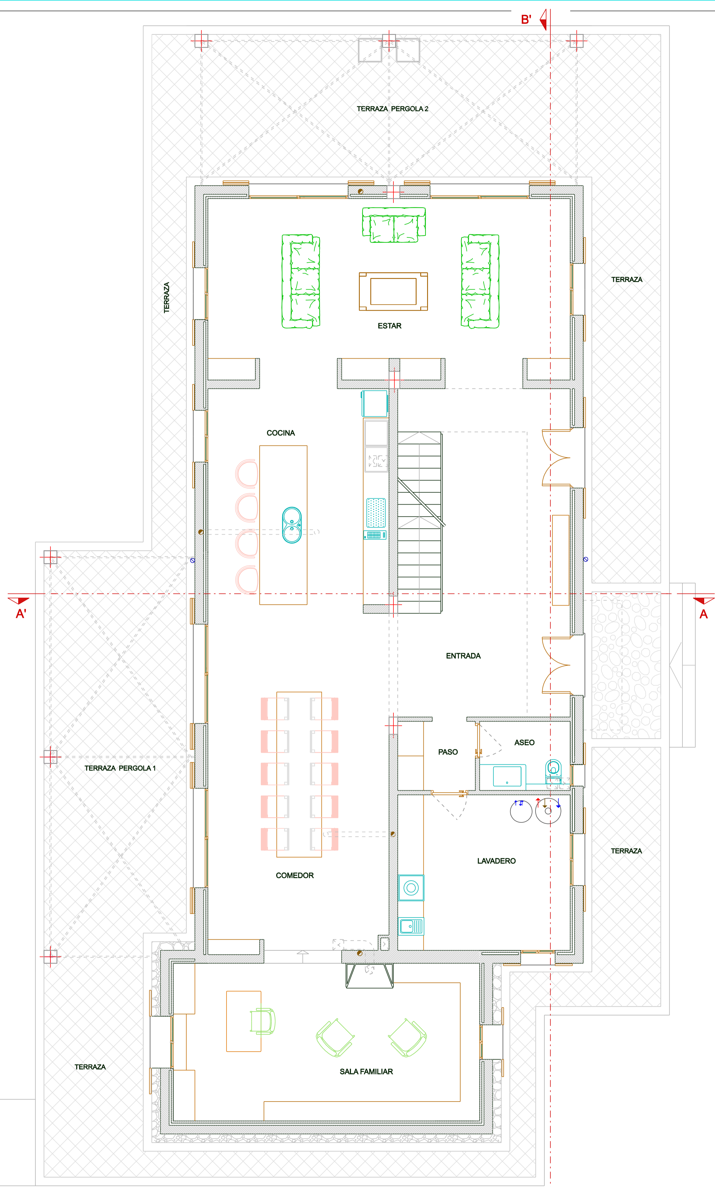
PLANTA BAJA DISTRIBUCION Sup. Construida Planta Baja.....196.11 m2
