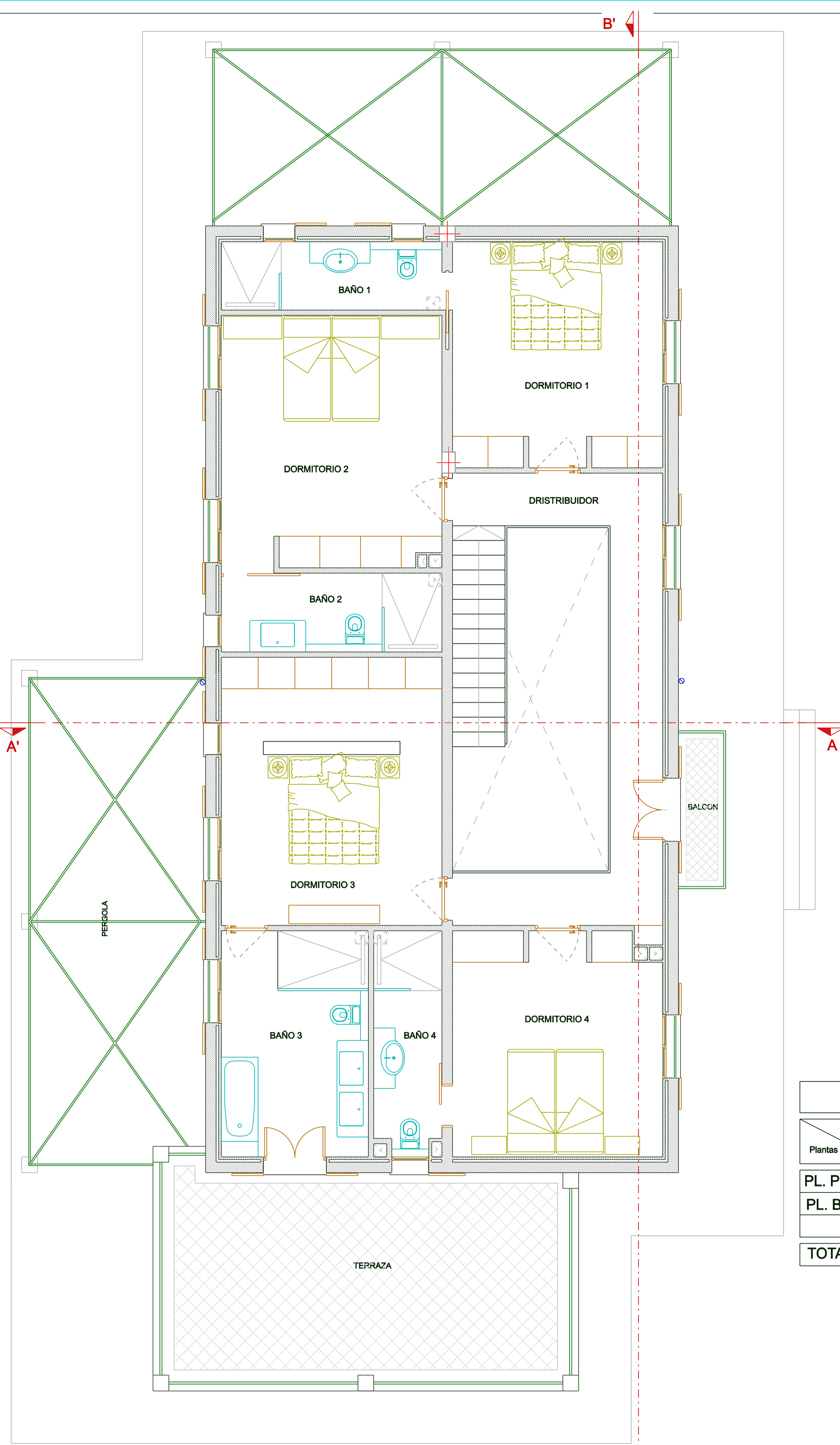
PLANTA PISO DISTRIBUCION Sup. Construida Planta Piso.....143.95 m2
