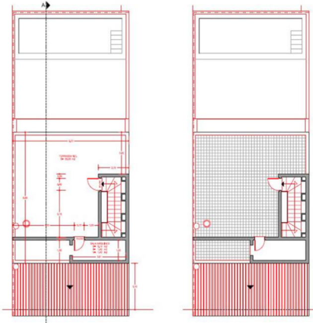
Planta pis 2n llocència 135/2017; cotes i superfícies e:1/100
