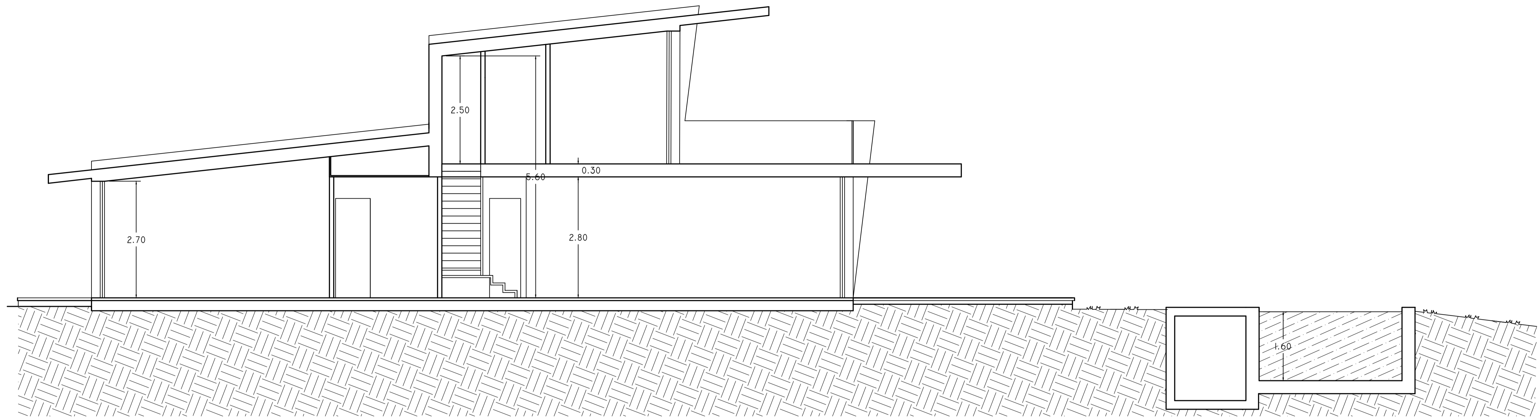
SECCIÓN A-A''
