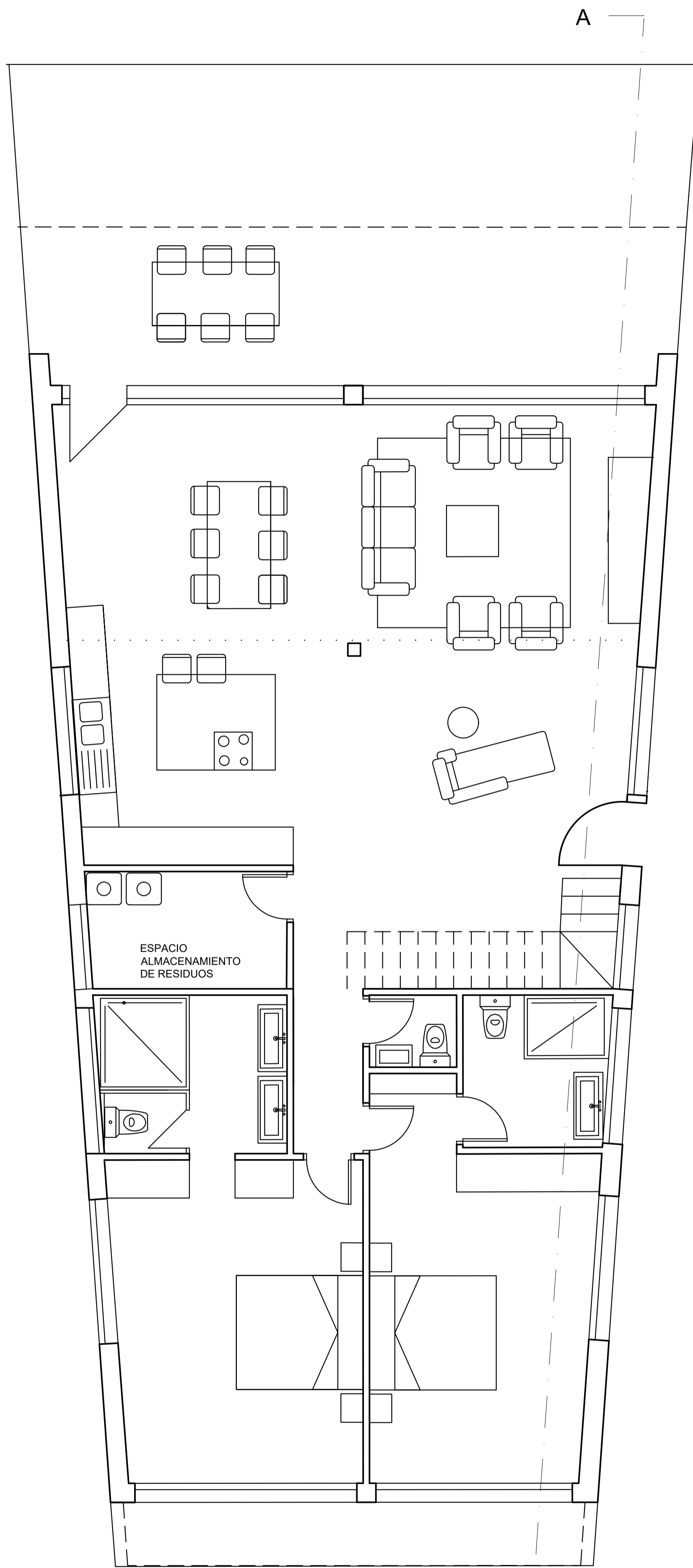
PLANTA BAJA
