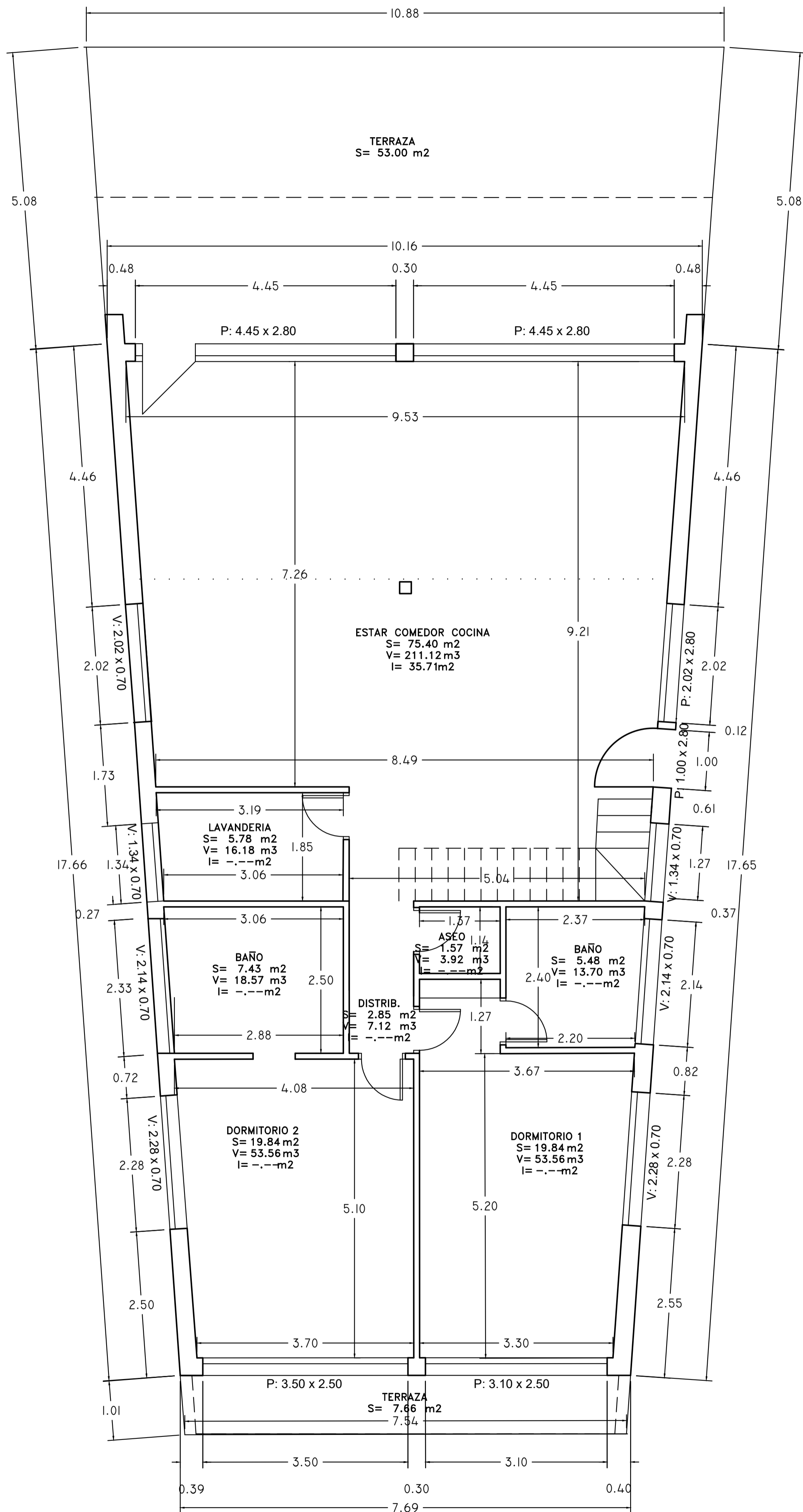
PLANTA BAJA
