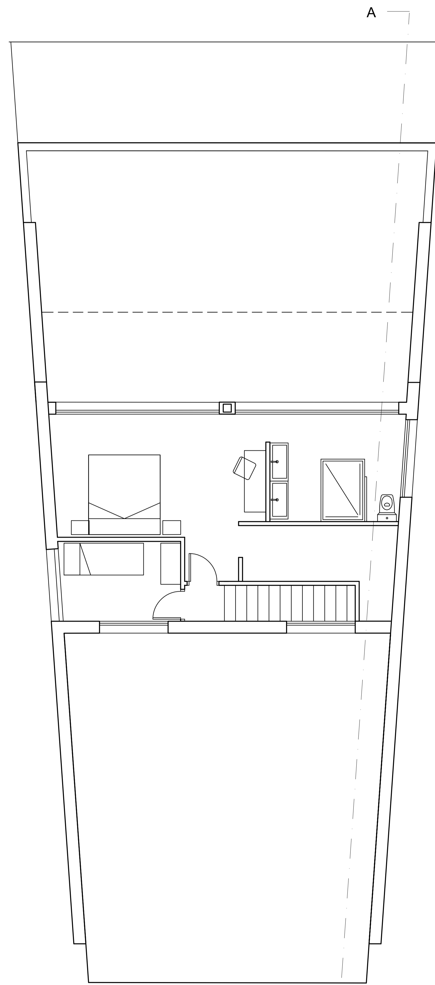
PLANTA PISO
