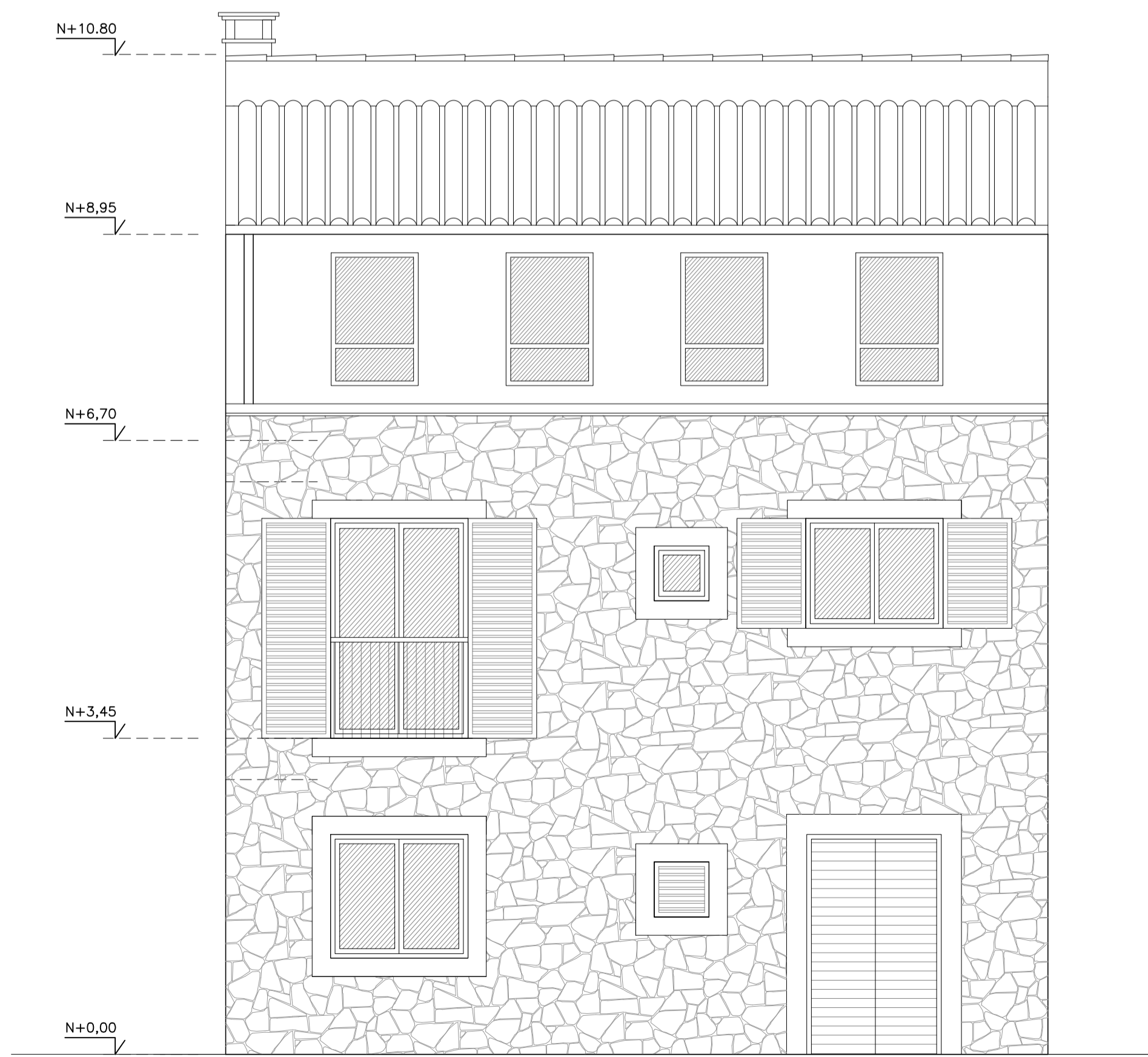
ALZADO FRONTAL
