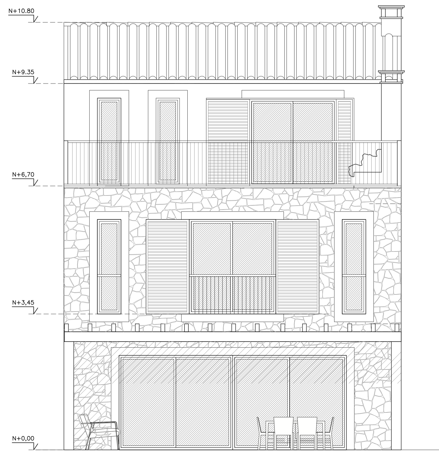
ALZADO POSTERIOR
