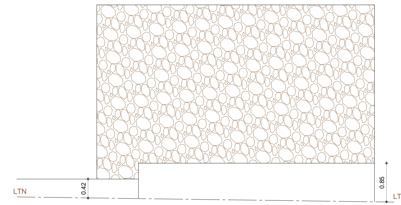
ALZADO POSTERIOR
