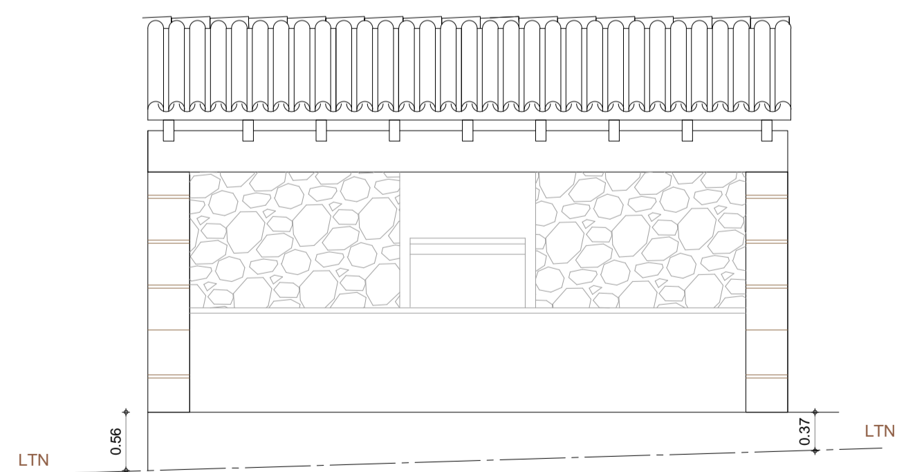
ALZADO FRONTAL
