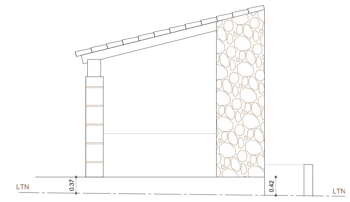
ALZADO LATERAL DERECHO
