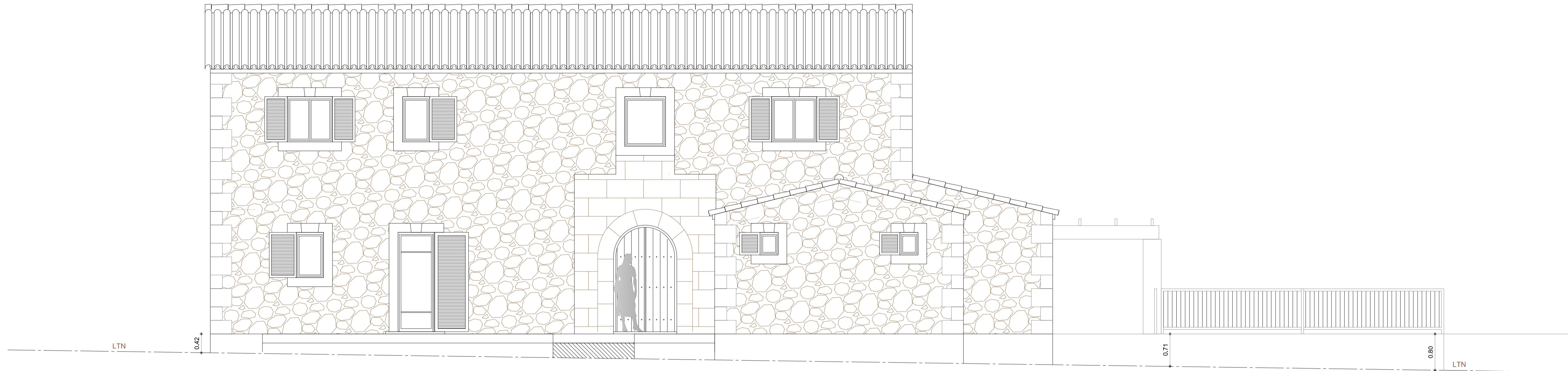
ALZADO FRONTAL
