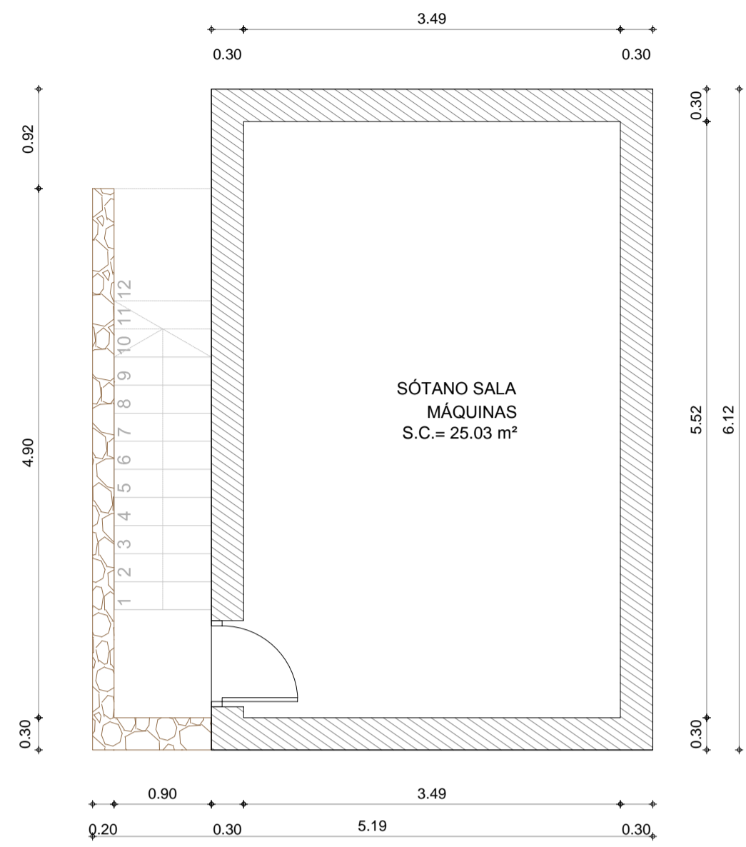
SOTANO SALA MÁQUINAS PISCINA
