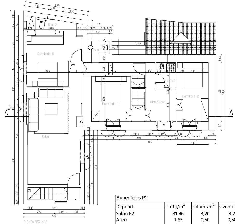
PLANTA SEGUNDA
