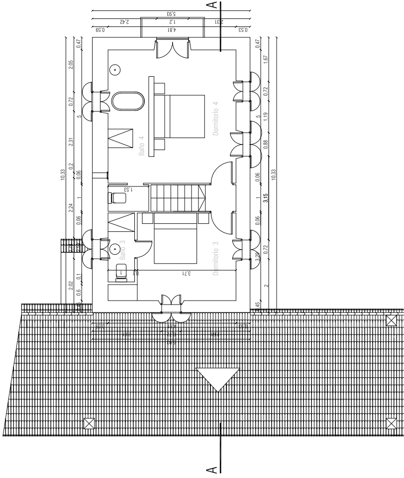
PLANTA TERCERA
